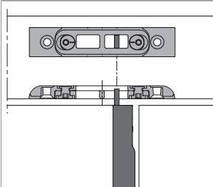
2-Flg. Tür mit 1 Riegel
